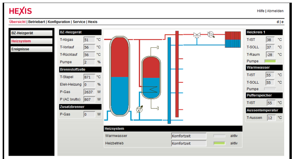
Abbildung 2 «Übersicht Heizsystem»-Seite (Quelle: Hexis AG)
